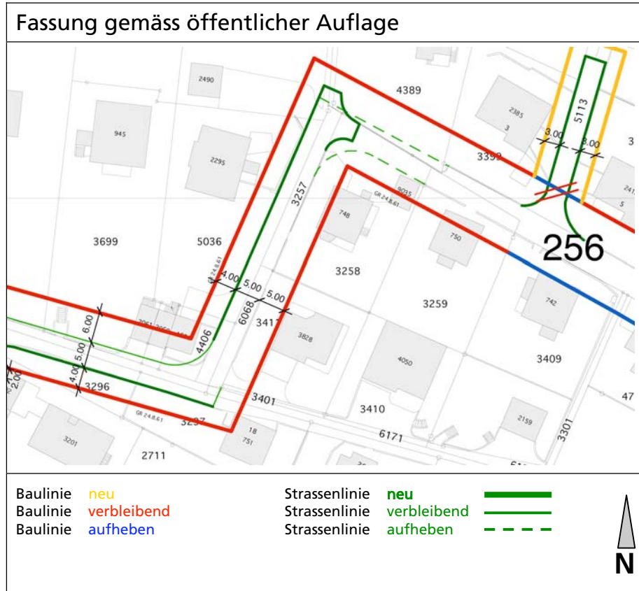
Planausschnitt 1 : 1'000
