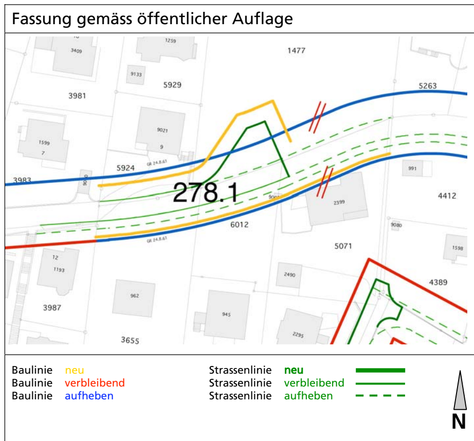
Planausschnitt 1 : 1'000
