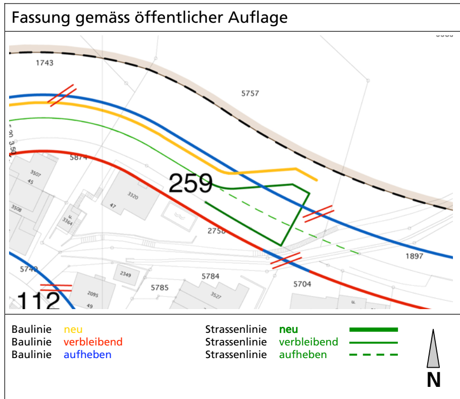
Planausschnitt 1 : 1'000
