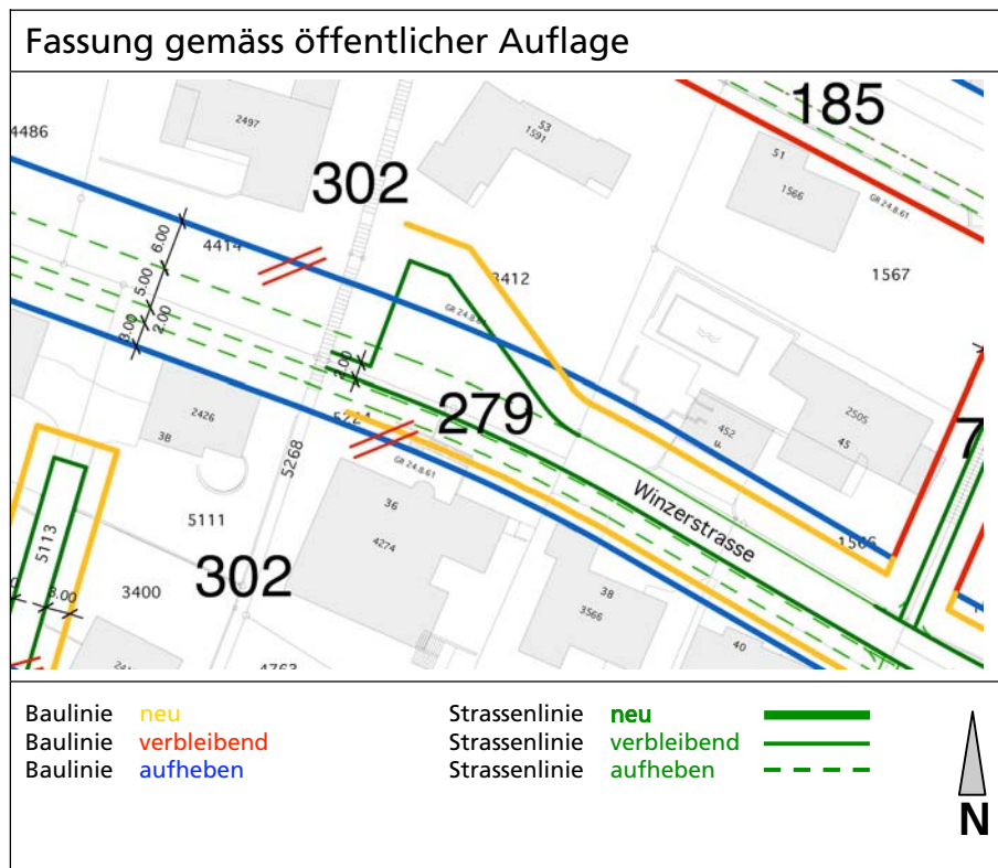
Planausschnitt 1 : 1'000
