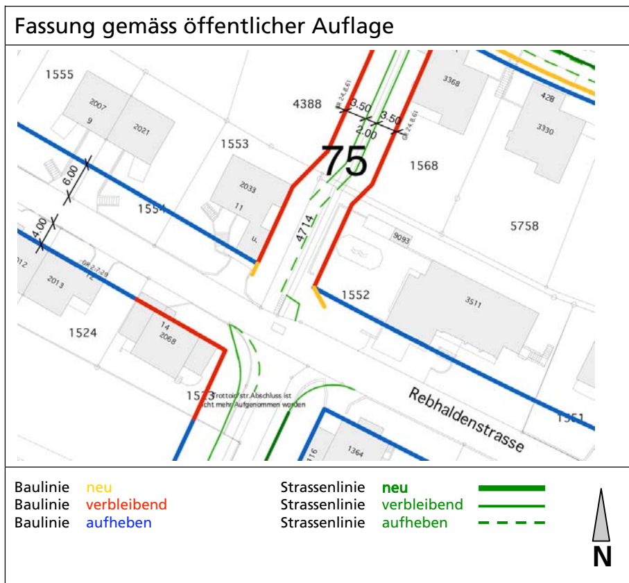
Planausschnitt 1 : 1'000
