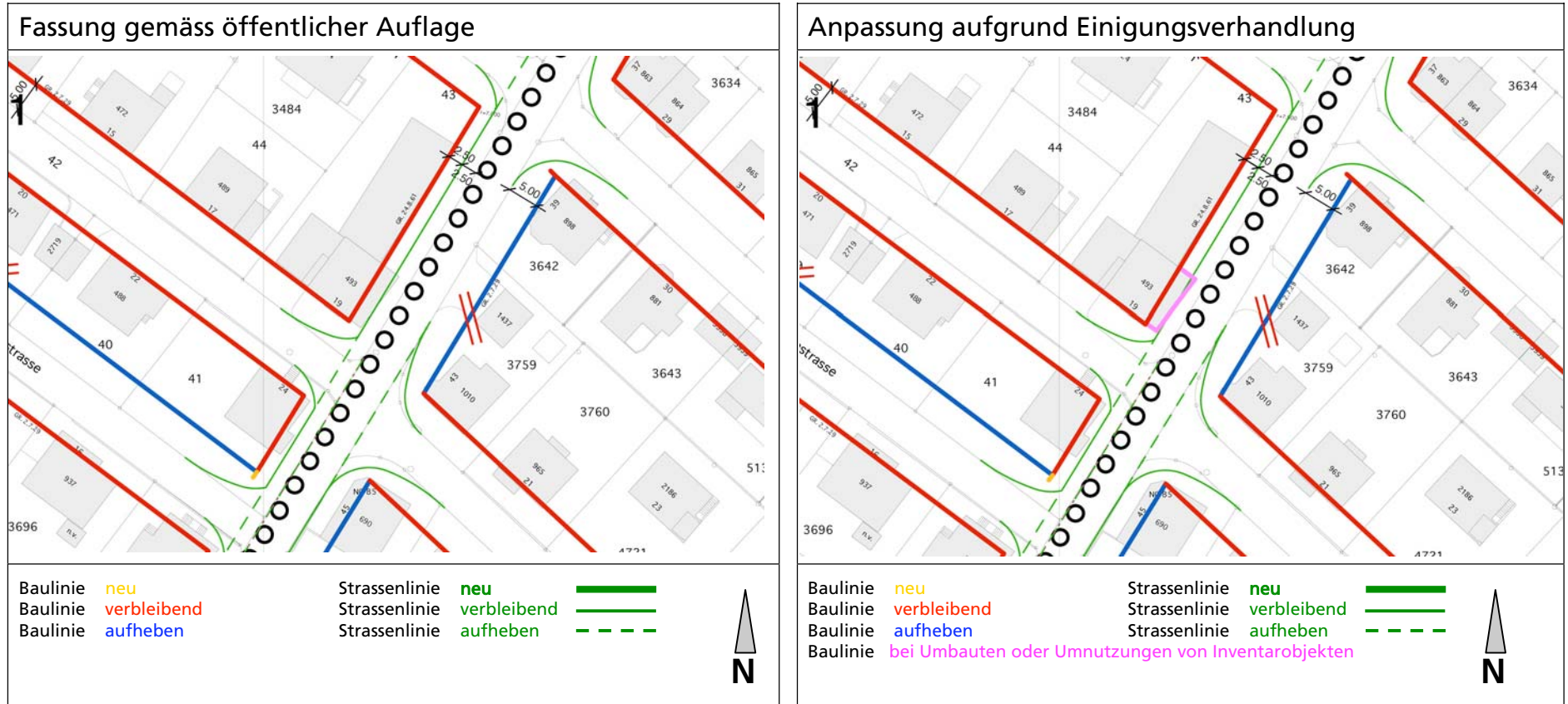
Planausschnitt 1 : 1'000
